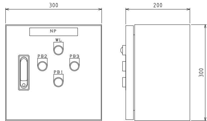
ターンテーブル 制御盤兼操作盤 (ケーブル長さ:5m)
