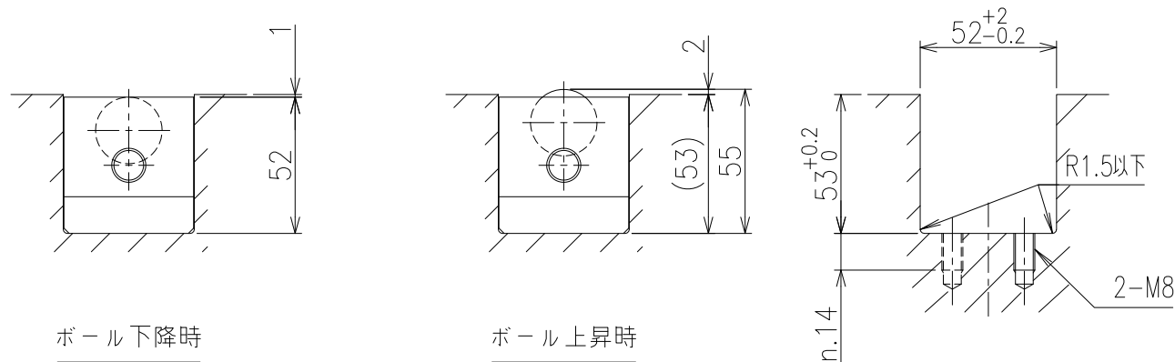
取付溝寸法図
