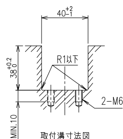
取付溝寸法図
