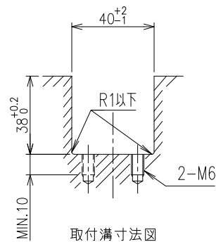
取付溝寸法図
